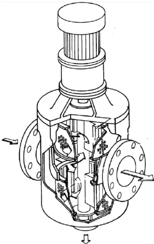
Strain-O-Matic painesiiviläsuodatin
