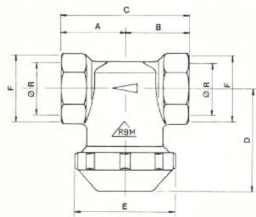
PN 16— DIN 2566 _ UNI 2223-2229
